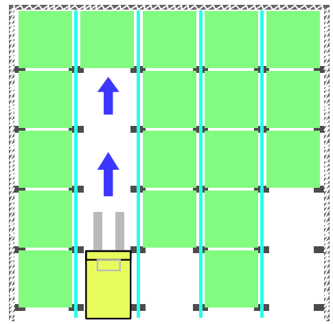
DRIVE-IN: dybdestablingsreol med adgang fra en side.
